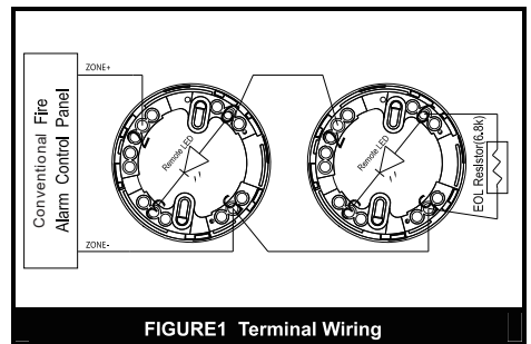
FIGURE1 Terminal Wiring
